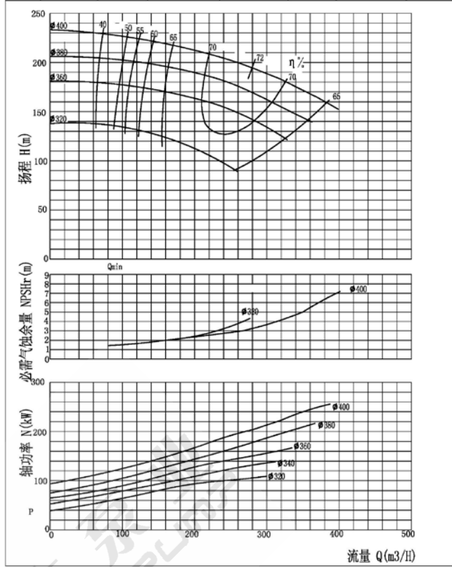
型号 100-400 转速 2950r/min 吸入口径 150mm 排出口径 100mm
