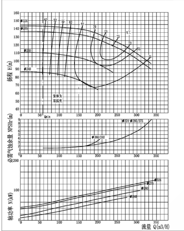
型号 100-315 转速 2950r/min 吸入口径 150mm 排出口径 100mm
