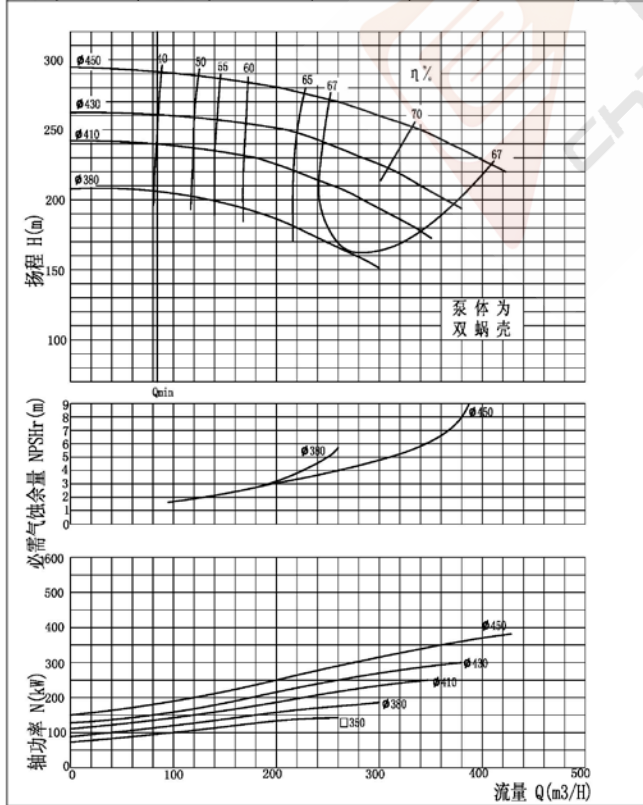
型号 100-450 转速 2950r/min 吸入口径 150mm 排出口径 100mm
