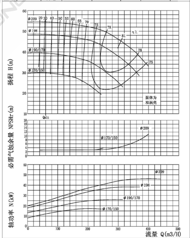
型号 150-200 转速 2950r/min 吸入口径 150mm 排出口径 150mm
